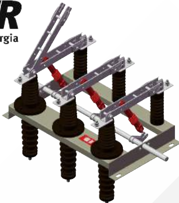
MODELO GV-06 SECCIONADORA TRIPOLAR , COM BUCHA DE PASSAGEM INTERNO/INTERNO ENTRADA INFERIOR OPÇÃO COM ENTRADA SUPERIOR
